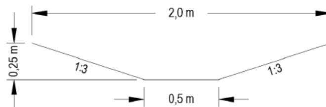
Figur 6. Tvärsektion på föreslagna svackdiken (WSP, Rev. 2024).
