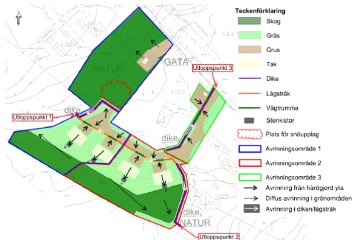
Figur 5. Systemlösning för dagvattenhantering (WSP, Rev. 2024).
